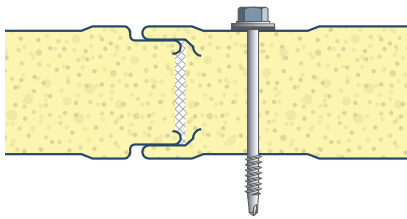
Zichtbare bevestiging enkelvoudige sluiting
