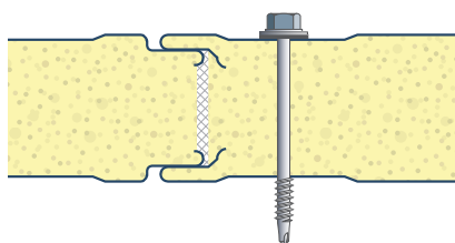
Zichtbare bevestiging enkelvoudige sluiting
