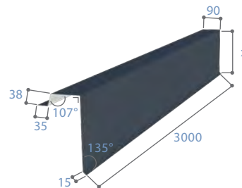
Windveer, x=afhankelijk van de paneel dikte
