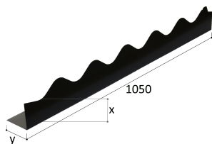
Isolatiebeschermingsprofiel
